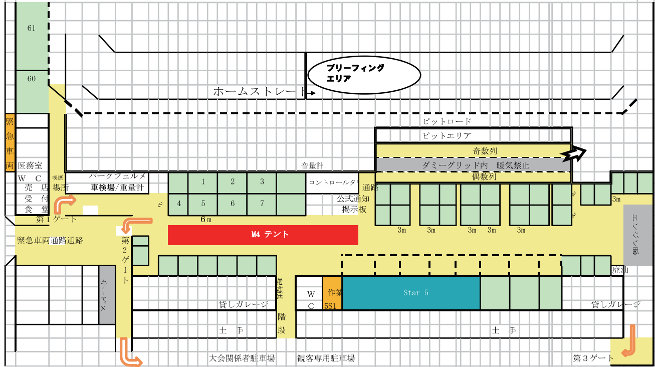
パドックレイアウト及び作業場・緊急車両配置図
